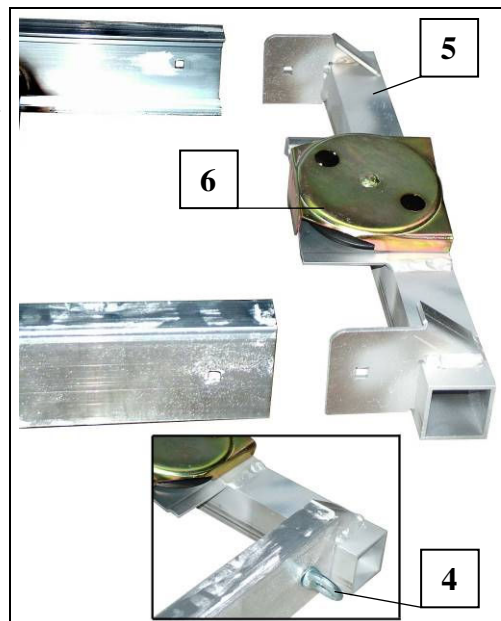
Fig. 20 Kopstuk monteren
