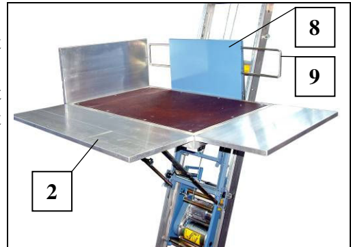
Fig. 53 Platformwanden verstellen
