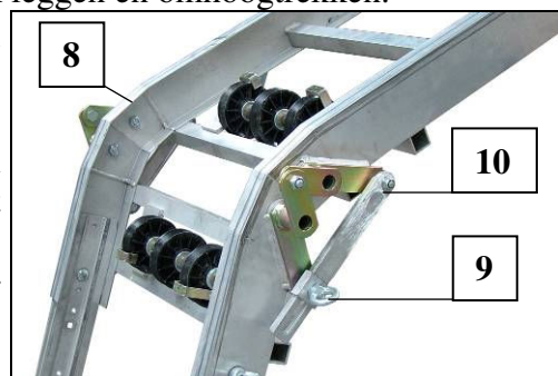
Fig. 22 Knikstuk instellen
