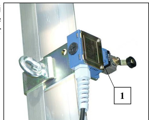
Fig. 10 Eindeloopschakelaar boven
