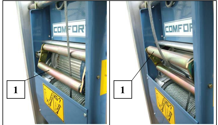
Fig. 11 Eindeloopschakelaar beneden
