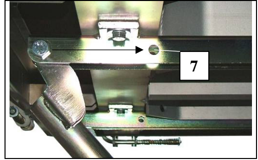
Fig. 52 Telescoopsteunen uitlijnen
