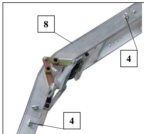
Fig. 21 Knikstuk monteren
